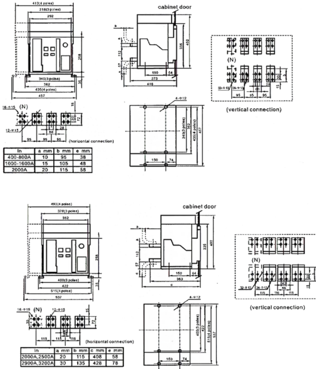
Diagrama No. 14 dimensiones y conexión (3200, 3200/4)
