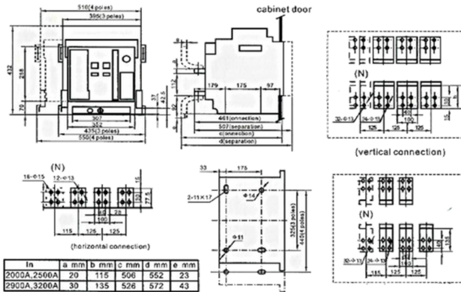
Diagrama No. 16 dimensiones y conexión tipo extracción (3200, 3200 / 4)
