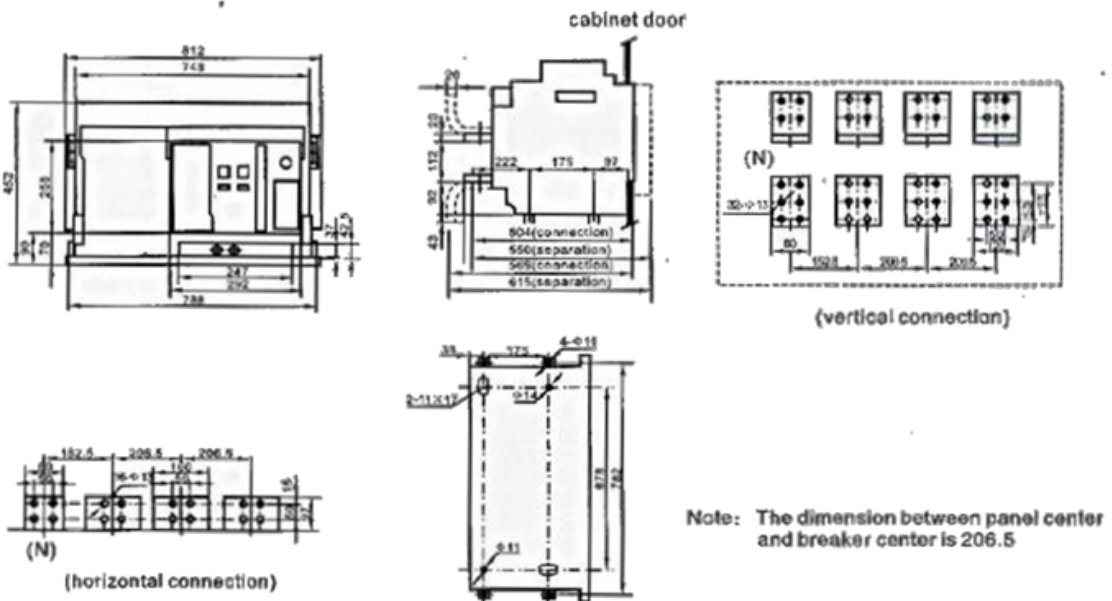
Diagrama 12 Dimensión y conexión del tipo de extracción (4000)
