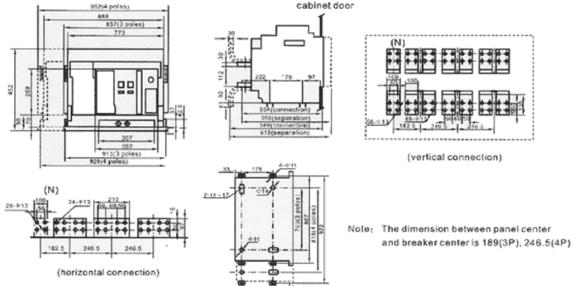
Diagrama 14. Dimensión y conexión del tipo de extracción (6300, 6300/4 In = 4000, 5000)
