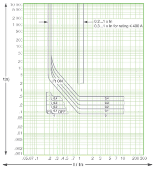
Protección contra defecto a tierra Planck V800
