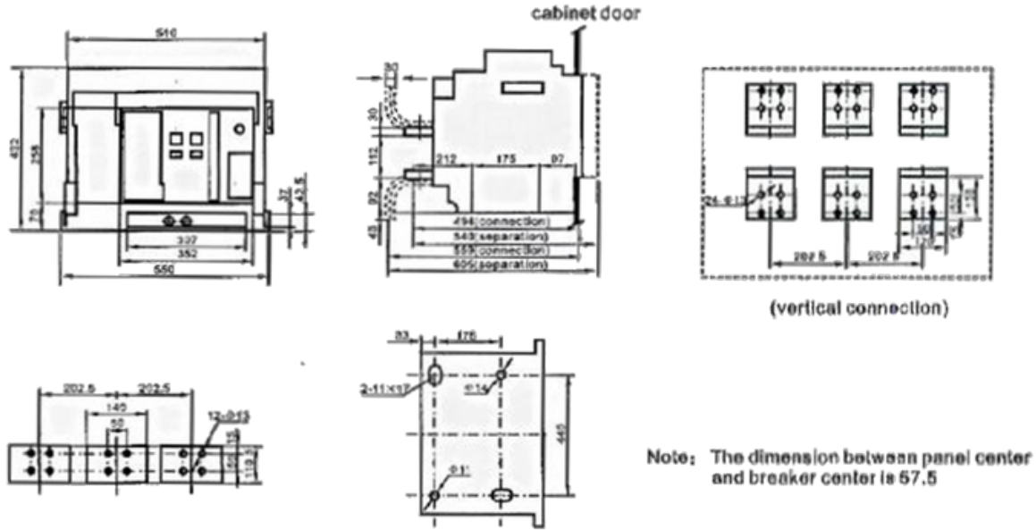
Diagrama 12 Dimensión y conexión del tipo de extracción (4000)
