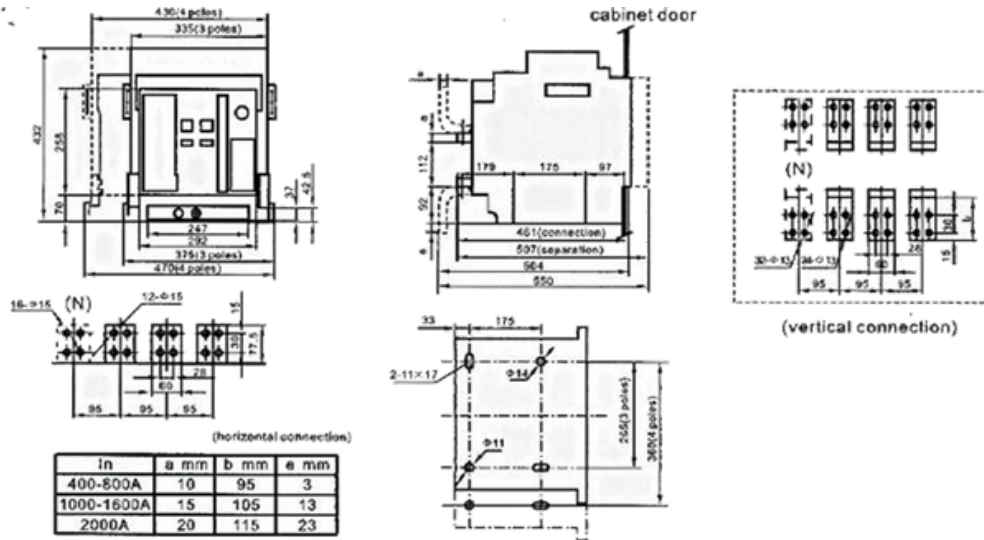
Diagrama No. 15 dimensiones y conexión tipo extracción (1000, 2000 / 3.4)
