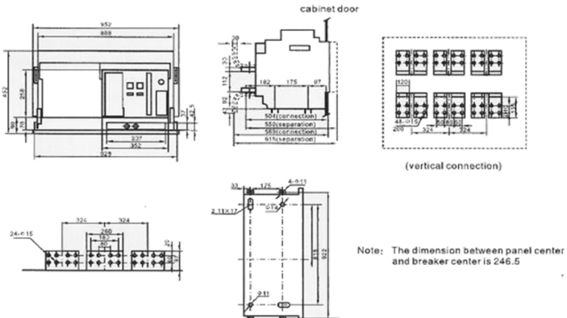
Diagrama 15 Dimensión y compuesto del tipo de extracción (6300 In = 6300 A)
