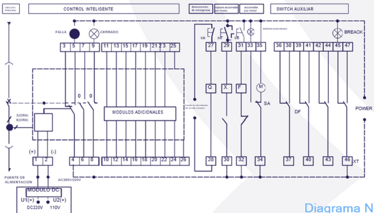
Diagrama de conexión para Master planck V(series)
